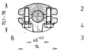
SCHNITT A - B
